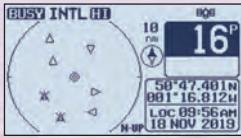
AIS Display
